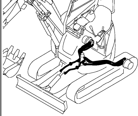
Fig. 65 油圧配管 (トラックフレーム) HYD. OIL PIPING (TRACK FRAME)
