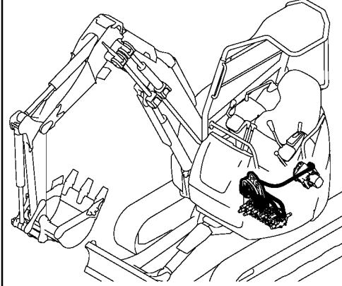
Fig. 62 油圧配管 (バルブ ~ スイベル) HYD. OIL PIPING (VALVE ~ SWIVEL)
