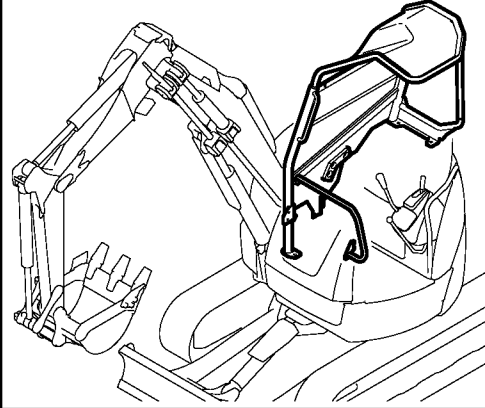
Fig. 40 キャノピー CANOPY
